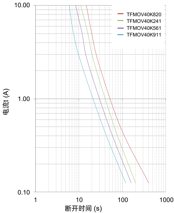
受限电流测试曲线 (UL 1449)
